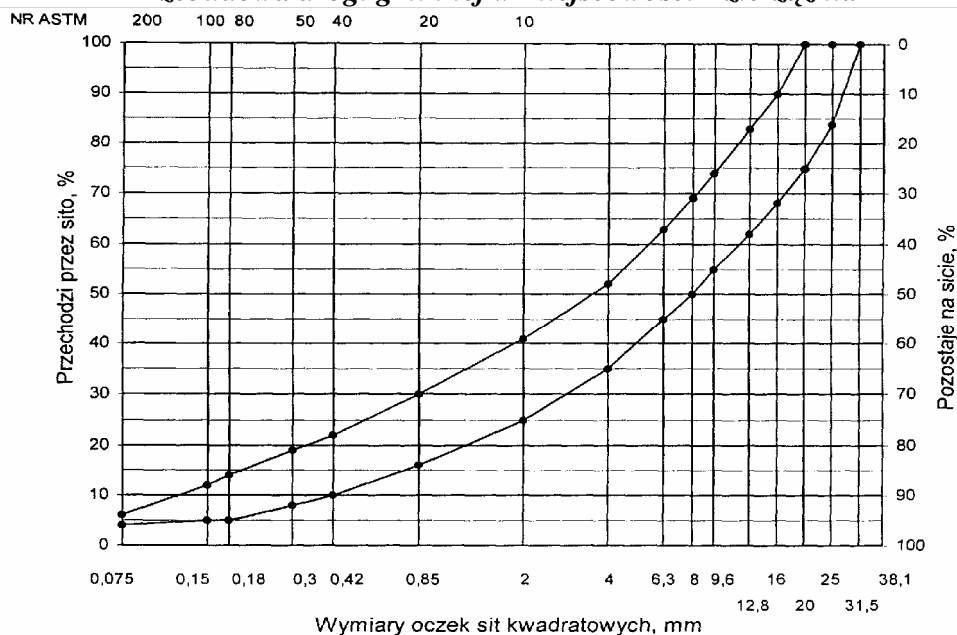
Rys. 12. Krzywe graniczne uziarnienia mieszanki mineralnej BA od 0 do 20 mm do warstwy wiążącej, wyrównawczej i wzmacniającej nawierzchni drogi o obciążeniu ruchem od KR3
