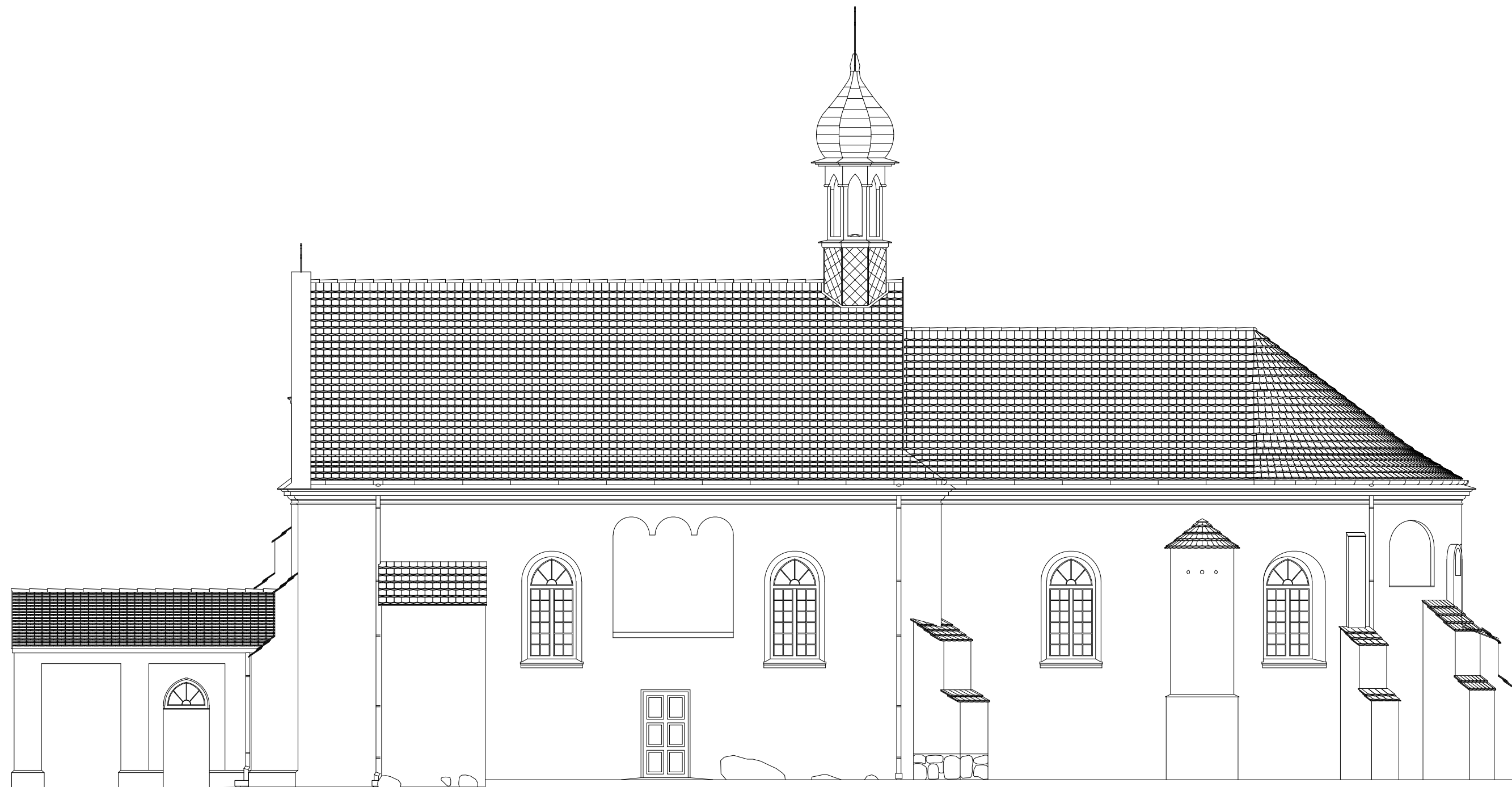
ELEWACJA POŁUDNIOWA
