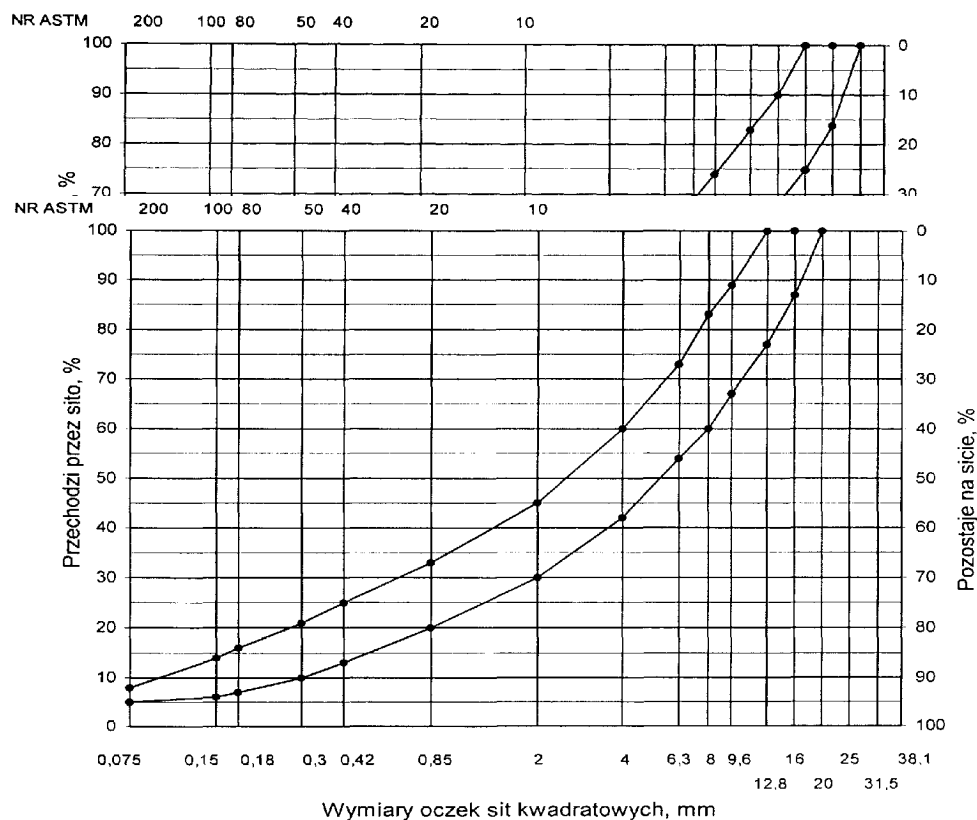
Rys. 13. Krzywe graniczne uziarnienia mieszanki mineralnej BA od 0 do 16 mm do warstwy wyrównawczej nawierzchni drogi o obciążeniu ruchem od KR3 do KR6
