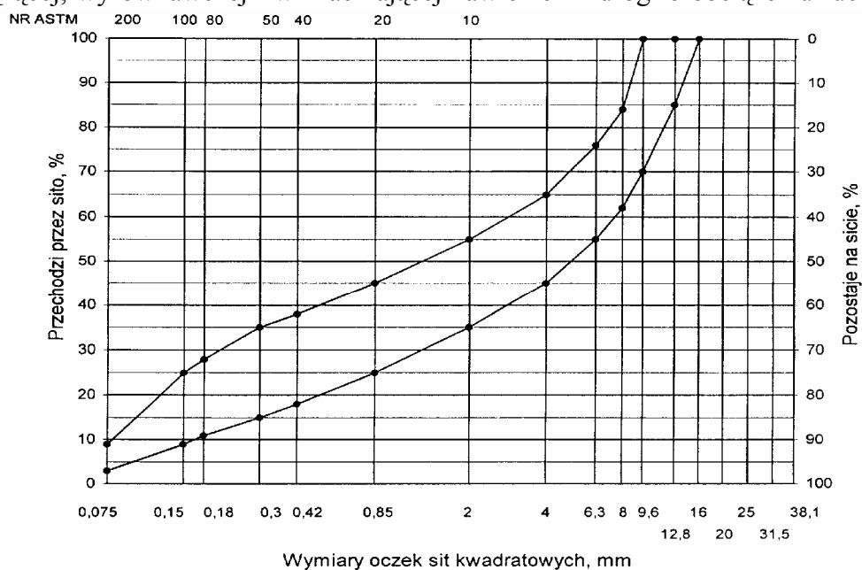
Rys. 9. Krzywe graniczne uziarnienia mieszanki mineralnej BA od 0 do 16 mm do warstwy wiążącej, wyrównawczej i wzmacniającej nawierzchni drogi o obciążeniu ruchem KR1 lub
